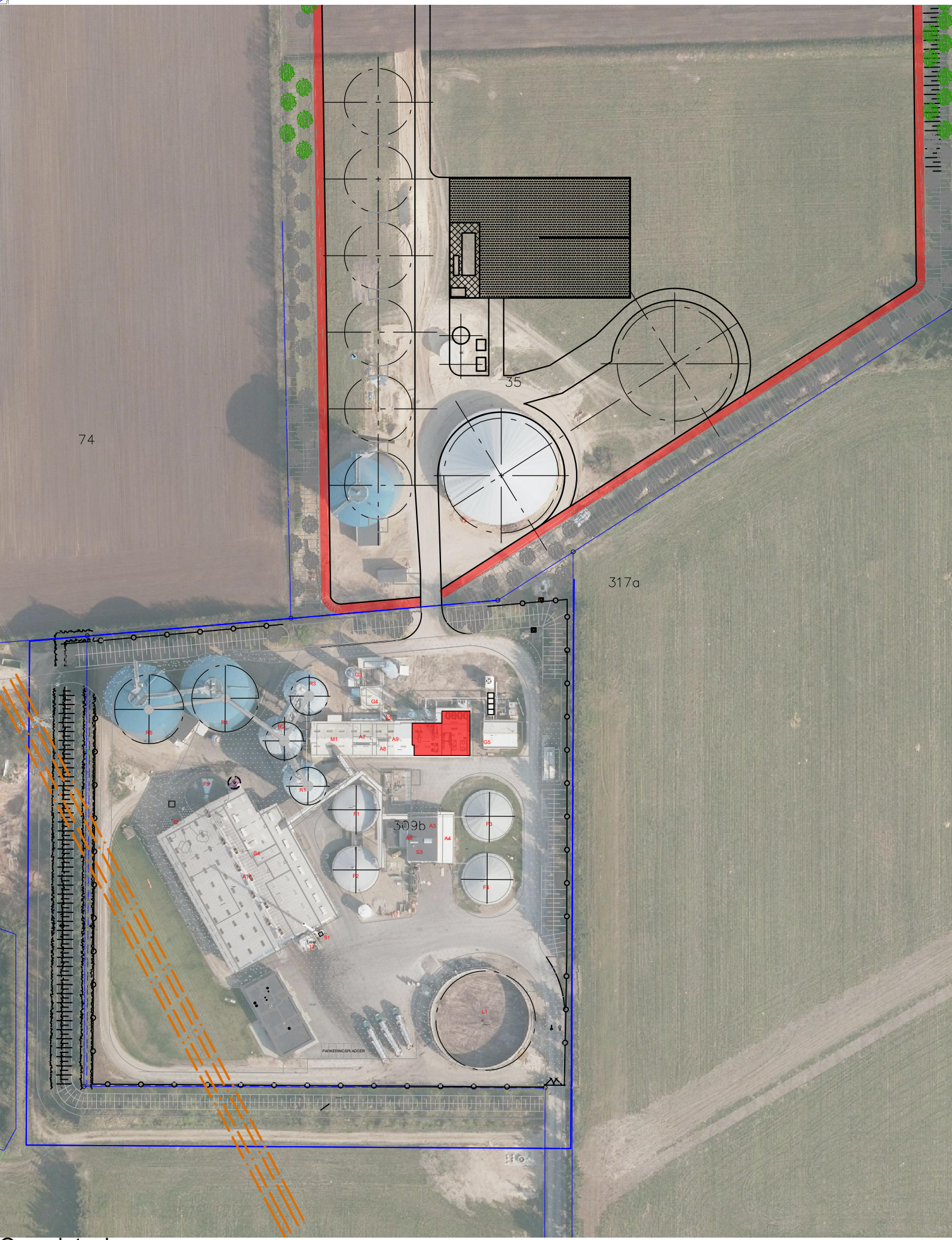
Oversigtsplan Mål: 1:1500
